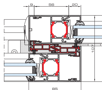
Przekrój przez środkowy słupek ruchomy
