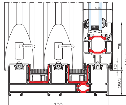
Notus trzy-torowy
