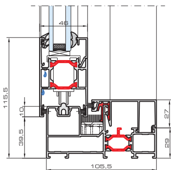
Notus jedno-torowy
