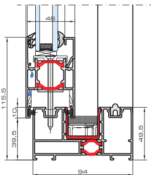
Notus dwu-torowy
